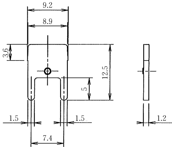
セット寸法例 Example of dimension for SET
