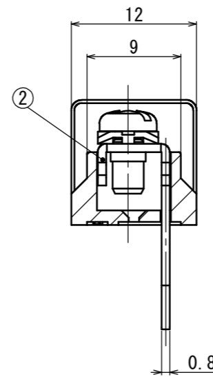
A-A 断面図 A-A Cross Section
