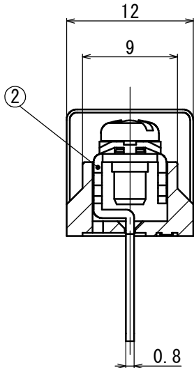
A-A 断面図 A-A Cross Section
