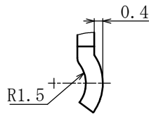
A 詳細図 (4/1) Detailed view A(4/1)
