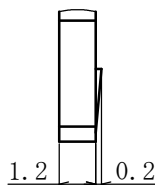
A 詳細図 (4/1) Detaild view(4/1)
