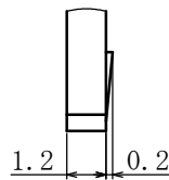
A 詳細図 (4/1) Detaild view(4/1)
