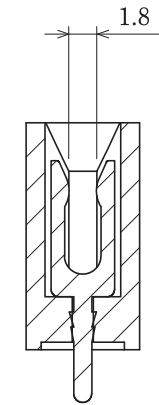
断面図 A-A スケール 2:1
