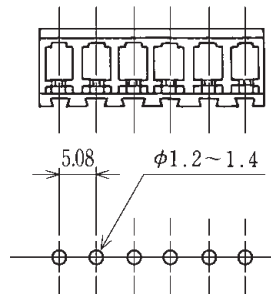
フロント基板寸法 PCB specifications
