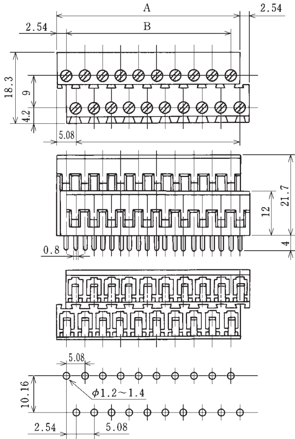
プリント基板寸法 PCB specifications
