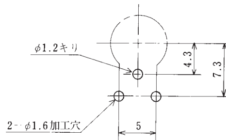
プリント基板加工図 Processing the printed board
