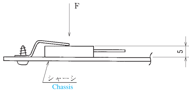
F9051トランジスタクリップ押付力 Pressing Force of F9051 Transistor Clip
