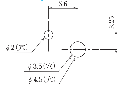
シャーシ加工例 Processing the chassis
