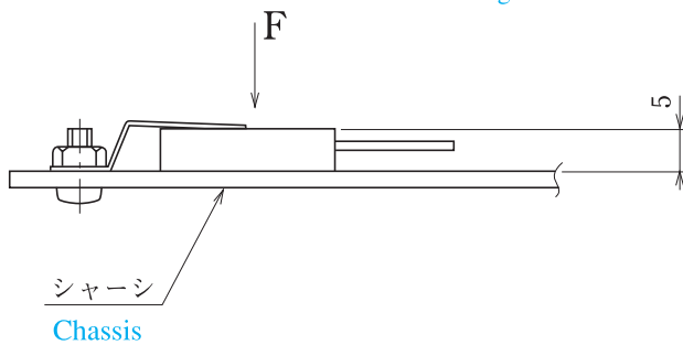
F9051H トランジスタクリップ押付力 Pressing Force of F9051H Transistor Clip
