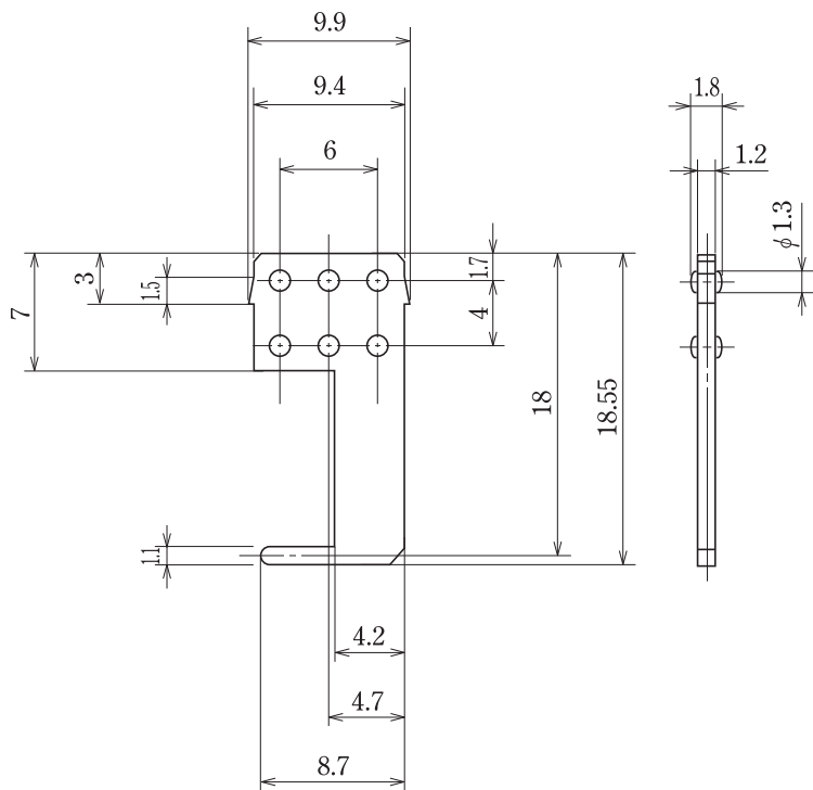
セット寸法例 Example of dimension for SET
