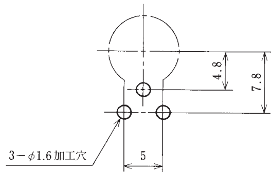
プリント基板加工図 Processing the printed board
