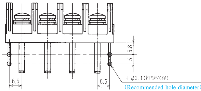
セット寸法例 Example of dimension for SET
