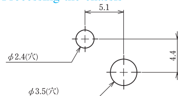
シャーシ加工例 Processing the chassis
