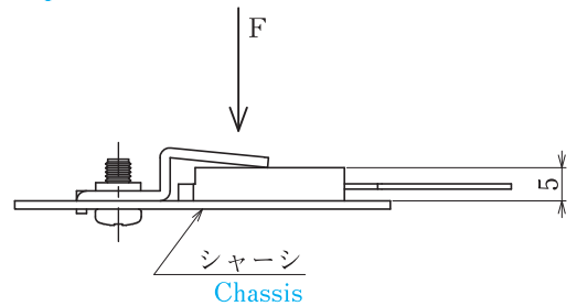
シャーシ加工例 Processing the chassis
