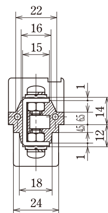
A-A 断面図
