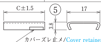
カバー止メ/ Cover retainer
