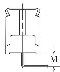
リード曲げ加工例 Example of a lead bent
