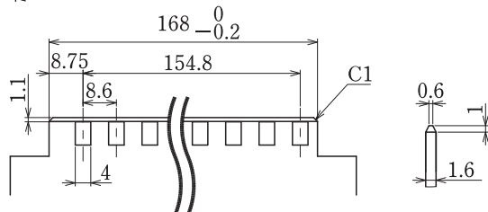
プリント基板仕様 PCB specifications
