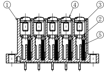
未結線時
