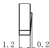
A 詳細図 (4/1) Detaild view A(4/1)
