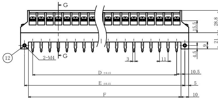
プリント基板穴寸法 PCB supecifications
