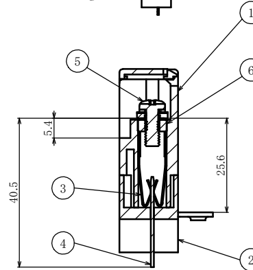
断面図G-G (1 / 1)
