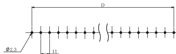
プリント基板穴寸法 PCB supecifications
