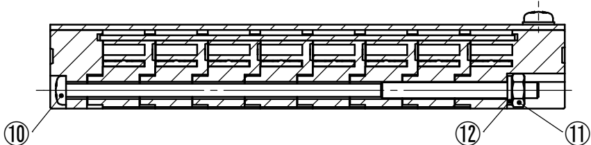
断面図 D-D
