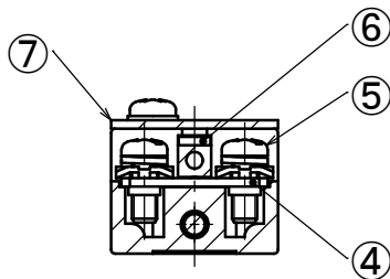
断面図 C-C
