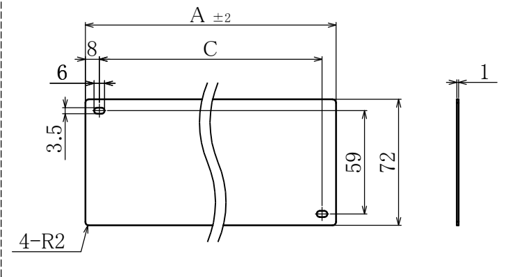
⑧カバー詳細図(1/3)
