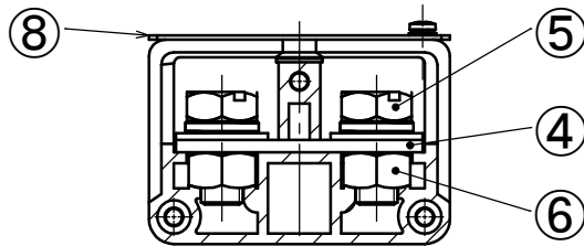
断面図 D-D
