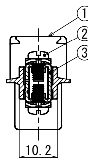
断面図A-A
