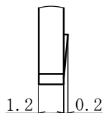
A 詳細図 (4/1) Detail view (4/1)
